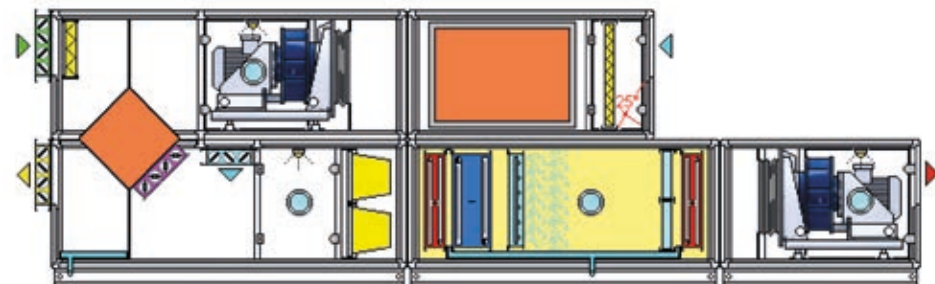
Fig. 3 UTA con recuperador estático y recirculación, batería de frío/calor y sección de humectación.
