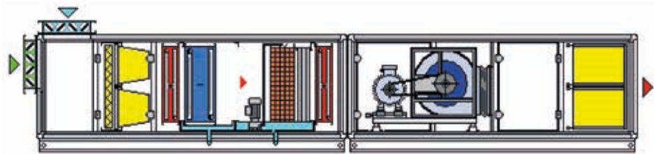
Fig. 2 UTA unidireccional con batería de FRÍO/CALOR, sección de humectación y filtro absoluto HEPA.
